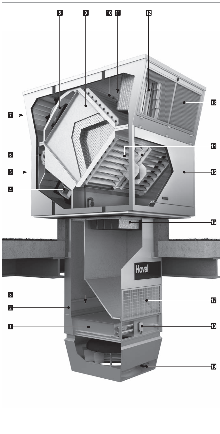
Рис. A2: Конструкция агрегата RoofVent® KH
