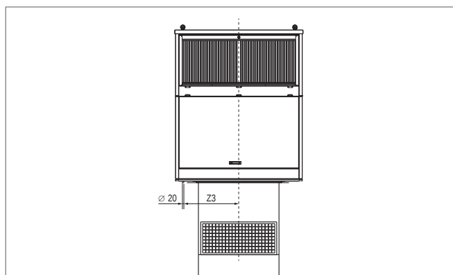
Табл. F4: Монтаж агрегатов RoofVent® на монтажное основание (размеры даны в мм)
