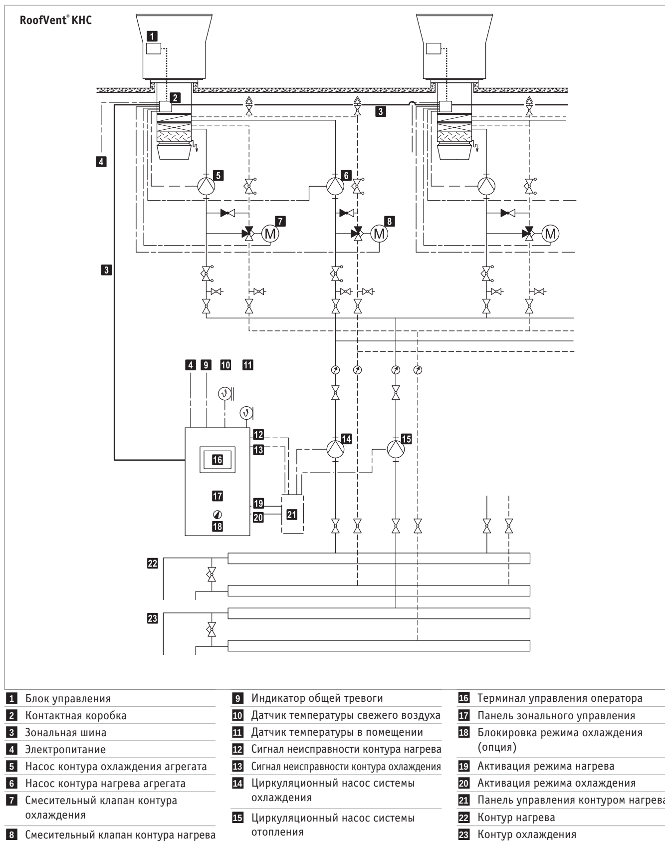
Табл. Е14: Схема гидравлической обвязки инъекционного типа для RoofVent® KHC
