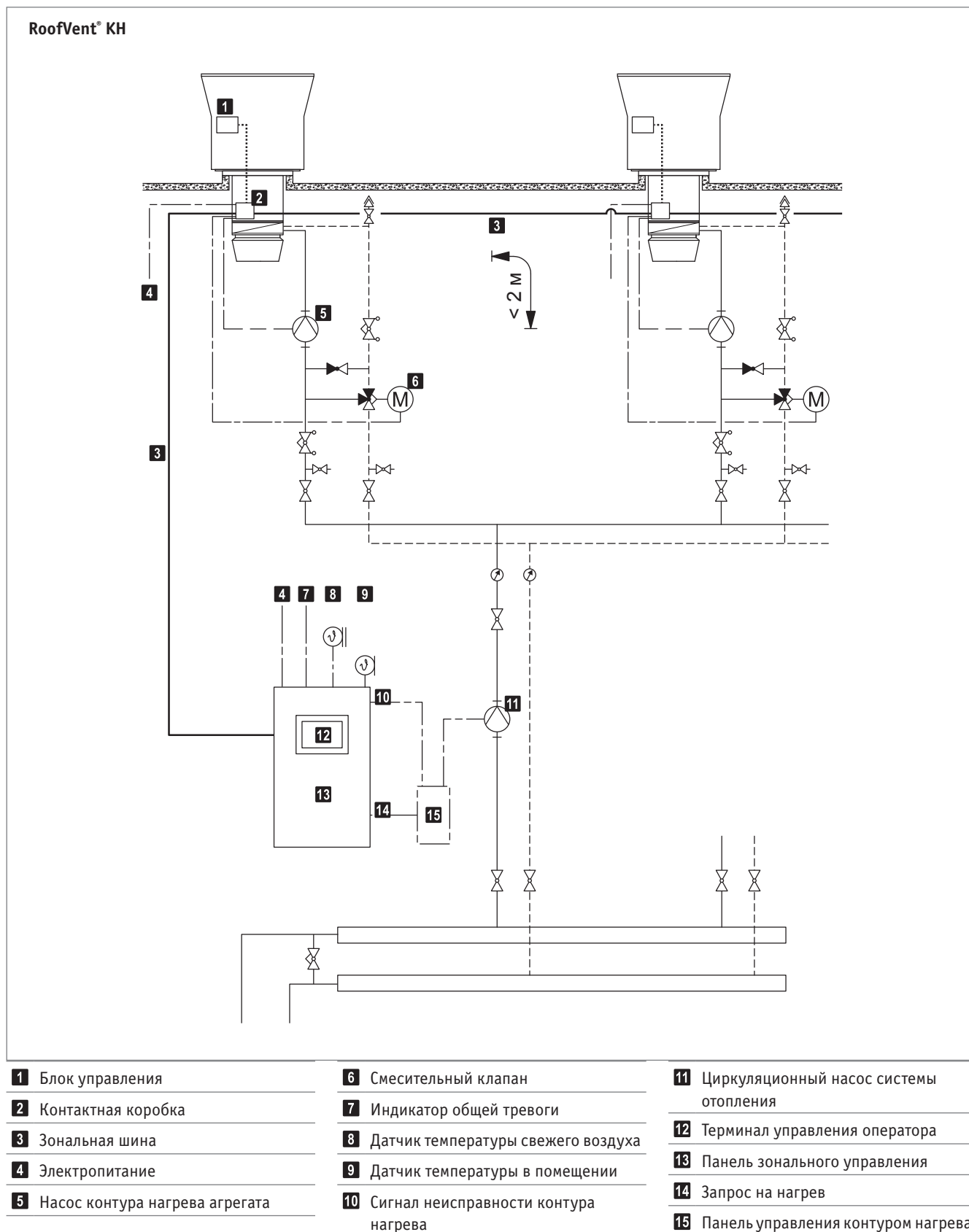
Табл. F11: Схема гидравлической системы девиационного типа агрегата RoofVent® KH
