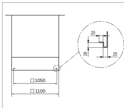
Рис. E5: Подключение воздуховода к агрегату
