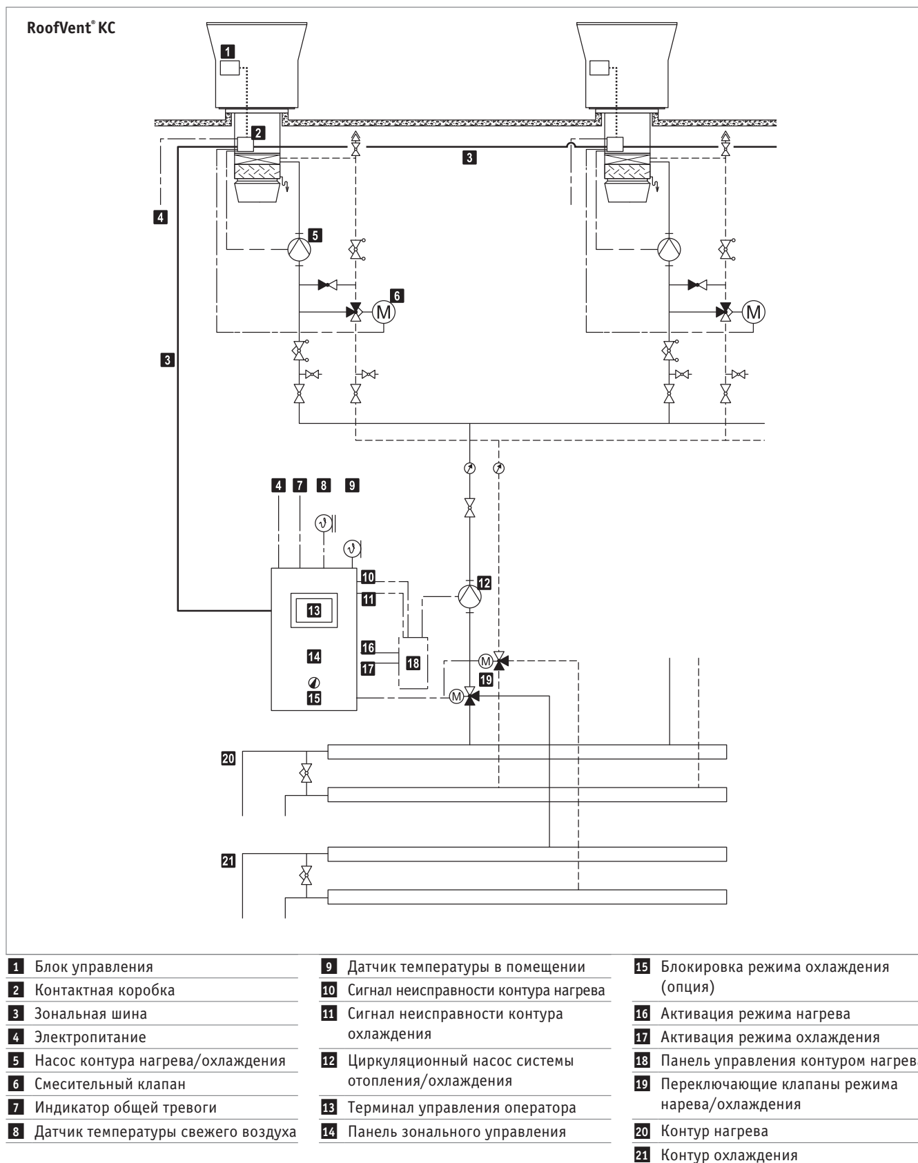
Табл. E13: Схема гидравлической обвязки инжекционного типа для RoofVent® KC
