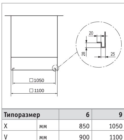
Рис. E4: Присоединительные размеры для приточного воздуховода (в мм)
