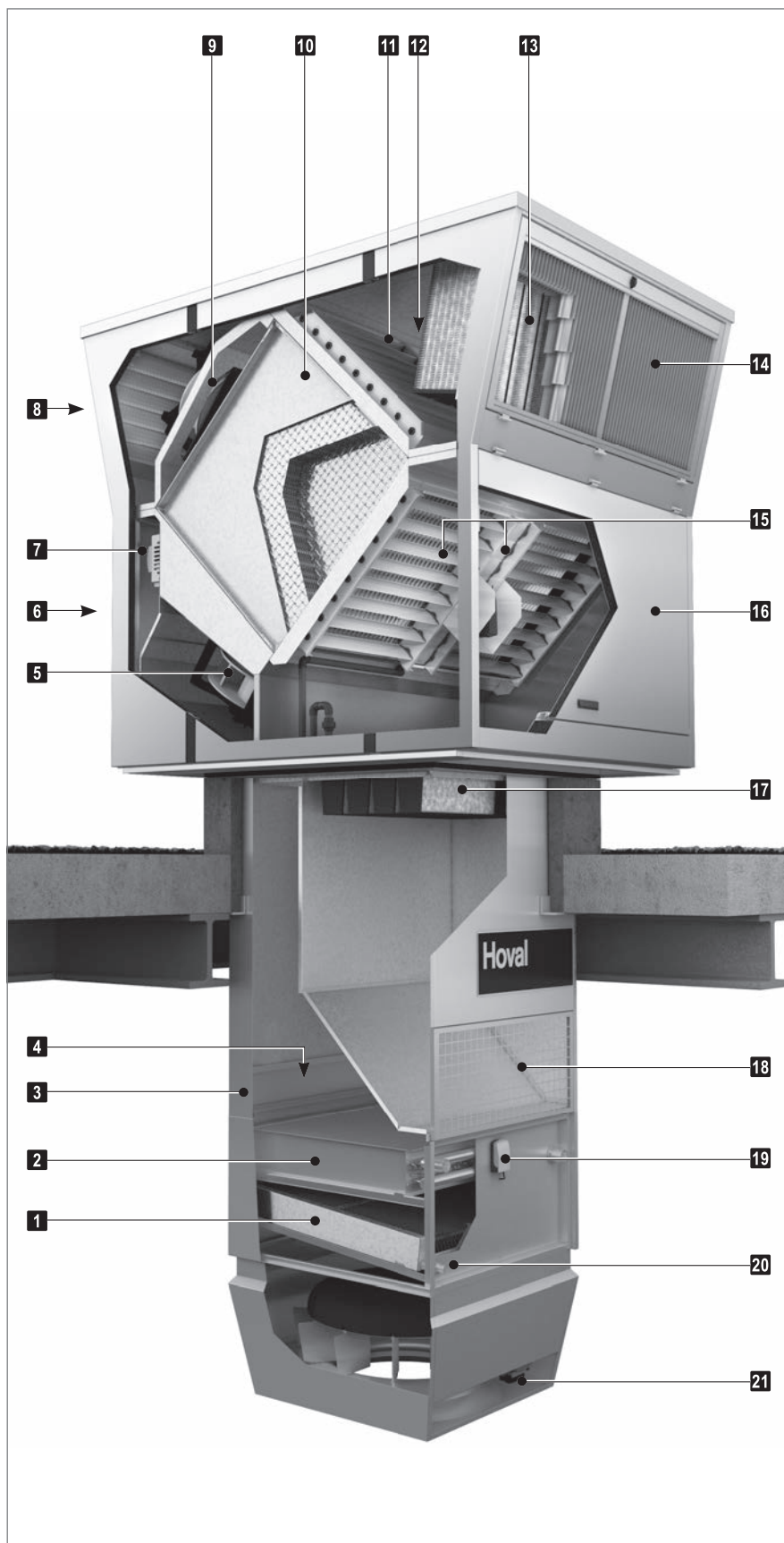
Рис. В2: Конструкция агрегата RoofVent® KC
