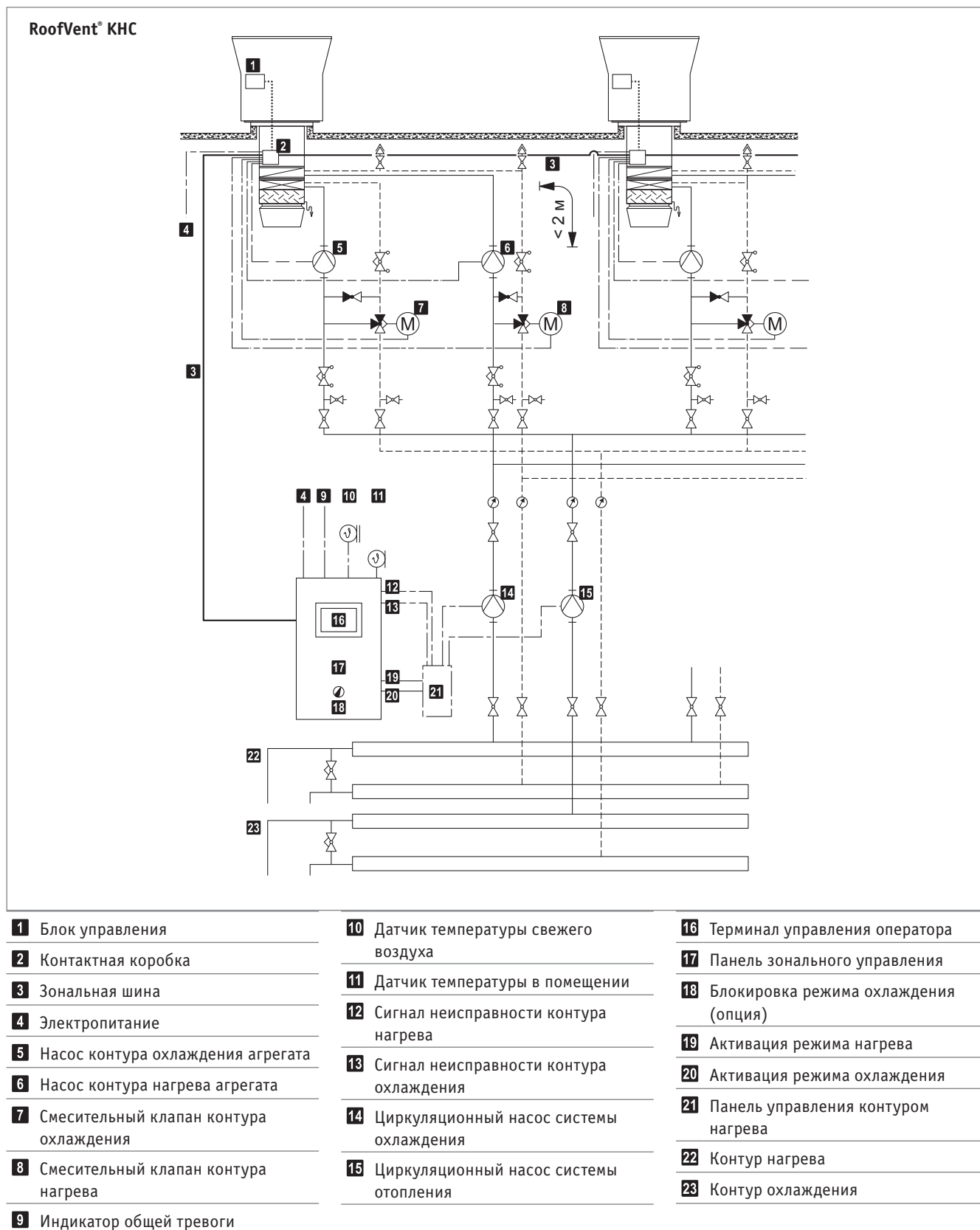
Табл. F13: Схема гидравлической системы девиационного типа агрегата RoofVent® KHC
