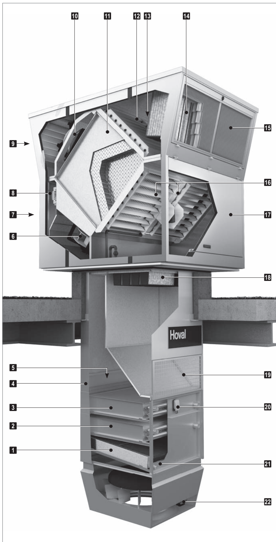
Рис. C2: Конструкция агрегата RoofVent® KHC
