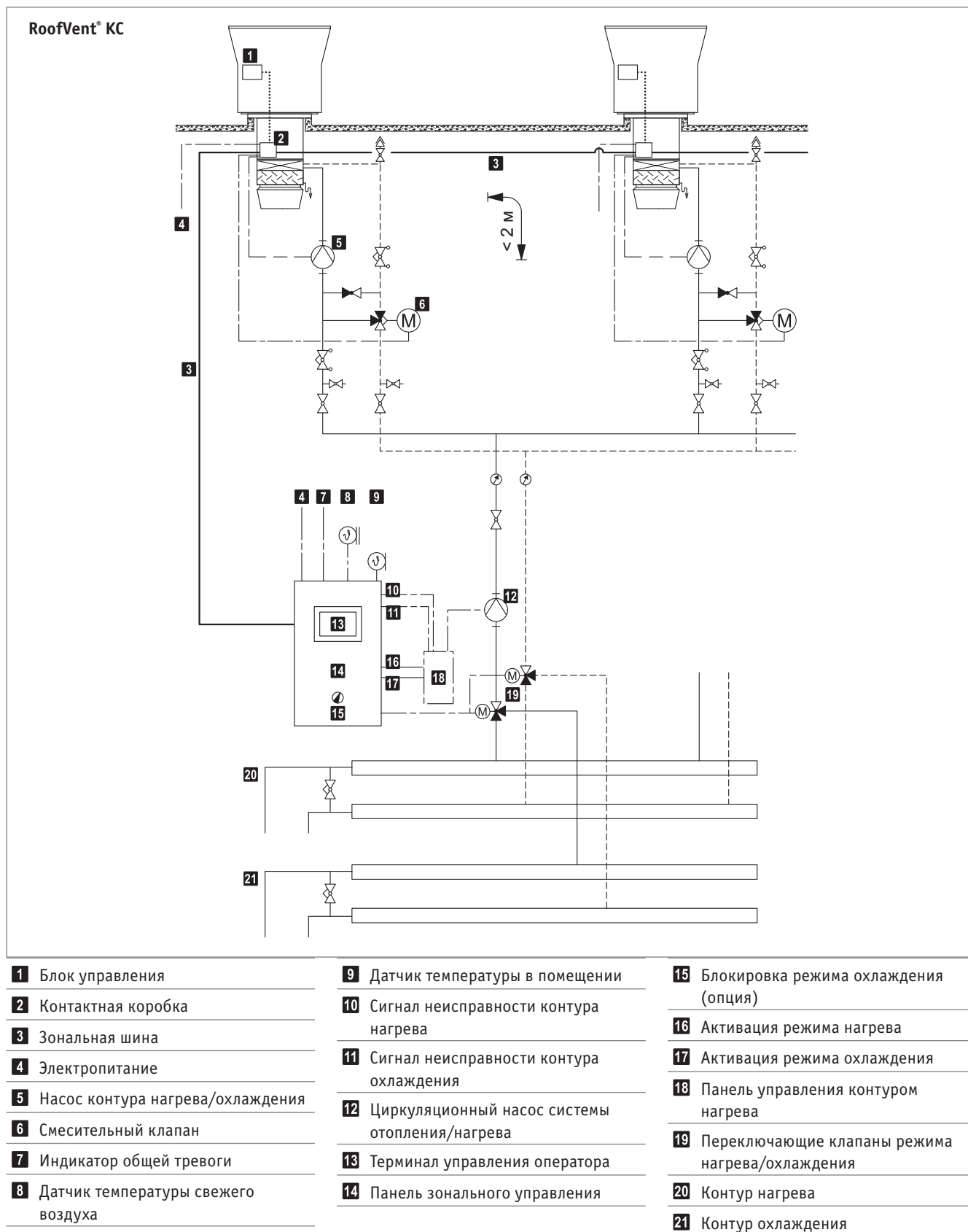
Табл. F12: Схема гидравлической системы девиационного типа агрегата RoofVent® KC
