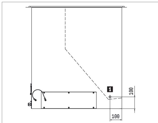
1 Патрубок для отвода конденсата от рекуператора G 3/4" (наружная резьба)
