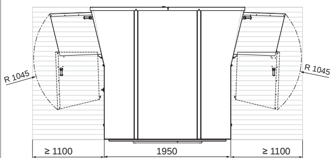
Табл. F2: Требования к сервисному пространству для проведения техобслуживания на крыше (размеры в мм)
