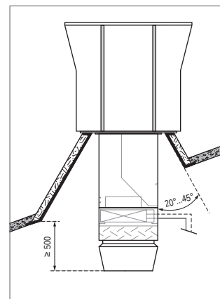
Рис. F2: Каркас с наклонными боковыми стенками конусообразной формы
