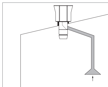
Табл. F9: Воздуховод вытяжного воздуха подсоединяется к соединительному модулю вместо решетки вытяжного воздуха
