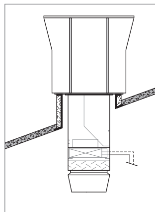
Рис. F1: Каркас с прямыми боковыми стенками
