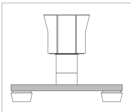
Рис. E3: Агрегат RoofVent с приточным воздуховодом и двумя воздухораспределителями Air-Injector
