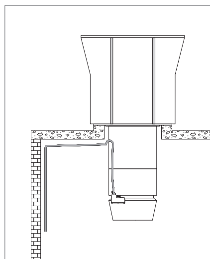
Рис. F3: Линия отвода конденсата
