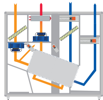
DanX XD Компактная приточно-вытяжная установка Dantherm с двойным рекуператором
