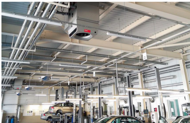
Автосалон Volkswagen, г. Краснодар Вентиляционные агрегаты
