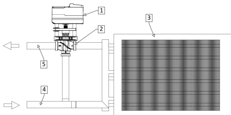
Подключение водяного теплообменника
