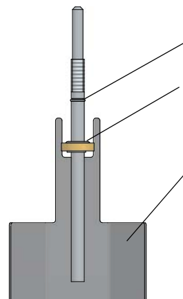
Двойное уплотнение электродов для парового цилиндра CY45/2 (SLE45/65)
