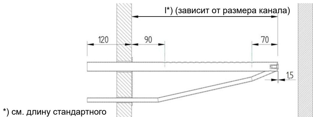
Горизонтальный монтаж в канале
